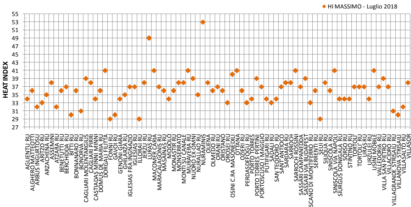
Figura 5 . HI massimo assoluto – Luglio 2018.
