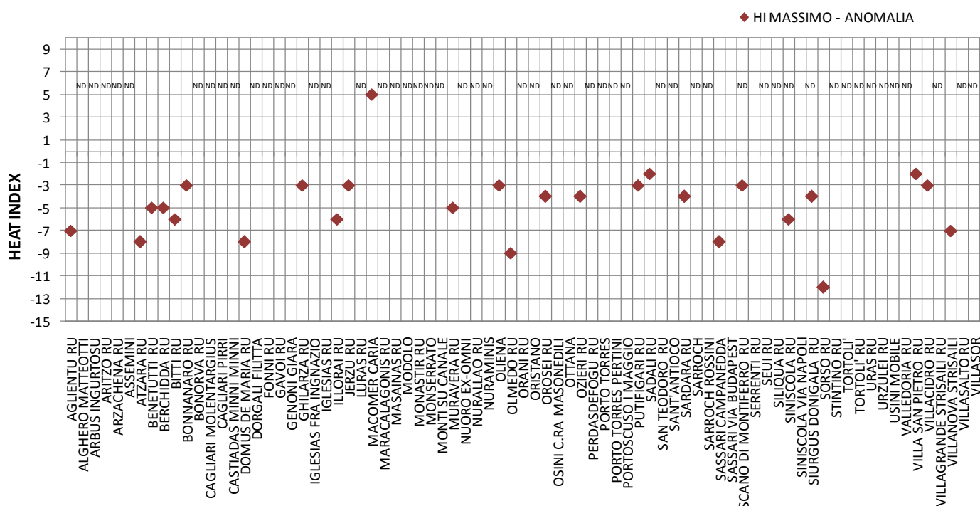
Figura 6. Anomalia dell'HI massimo assoluto rispetto alla media pluriennale di luglio 1995-2014.
