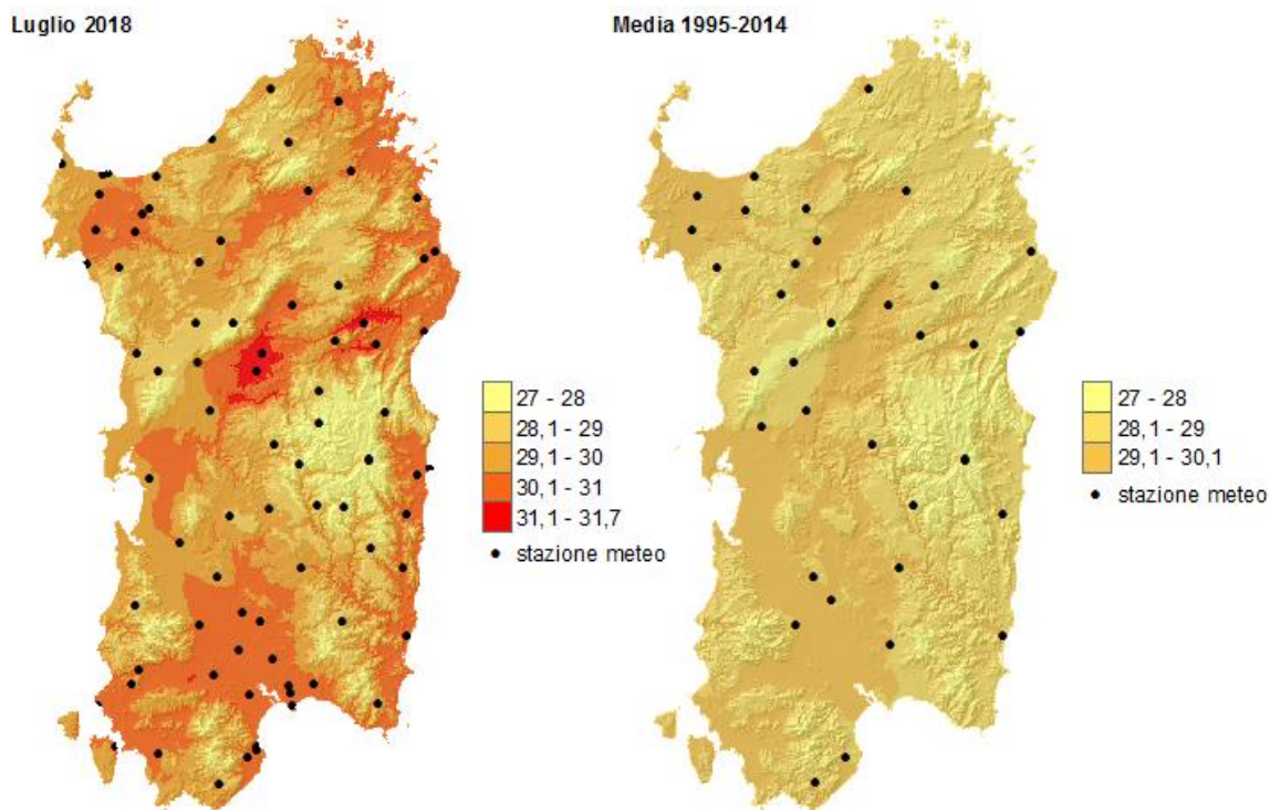
Figura 1. HI medio e raffronto con i valori medi del periodo 1995-2014 – Luglio 2018.
