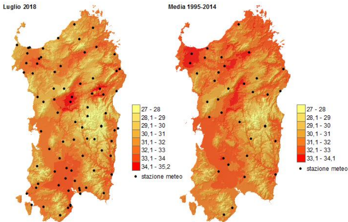
Figura 2. HI massimo e raffronto con i valori medi del periodo 1995-2014 – Luglio 2018.
