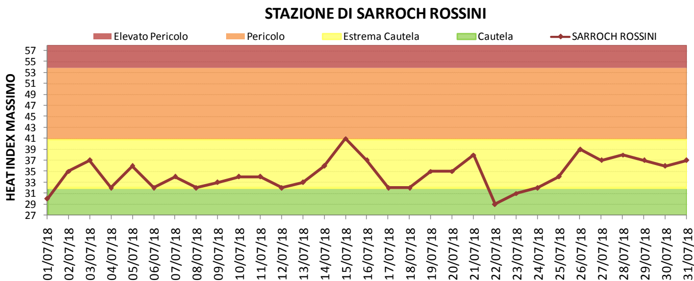
Figura 13. HI massimo giornaliero – Stazione di Sarroch Rossini.
