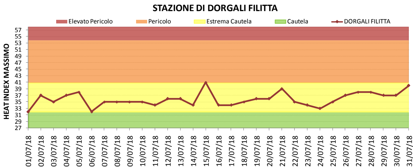
Figura 7. HI massimo giornaliero – Stazione di Dorgali Filitta.
