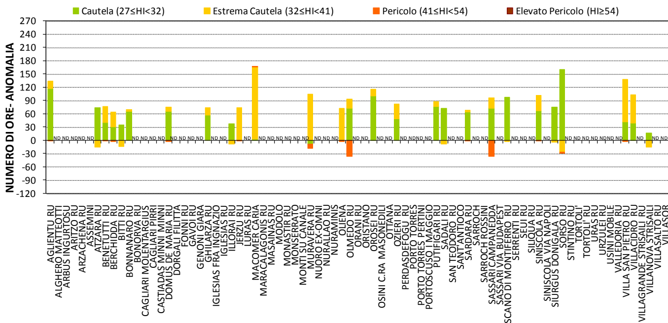
Figura 4. Anomalia delle ore con HI nei diversi livelli di disagio rispetto alla media pluriennale di luglio 1995-2014.
