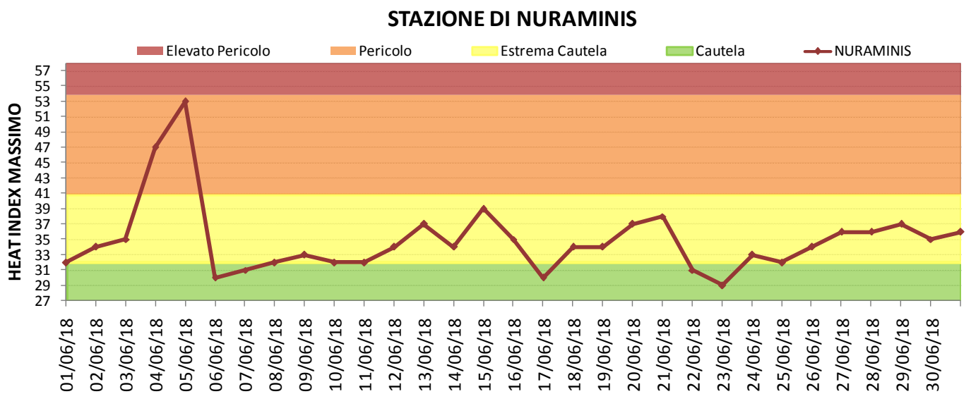
Figura 10. HI massimo giornaliero – Stazione di Nuraminis.
