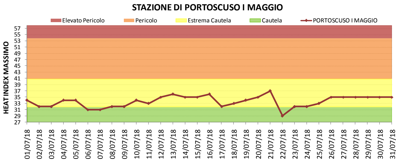
Figura 12. HI massimo giornaliero – Stazione di Portoscuso I Maggio.
