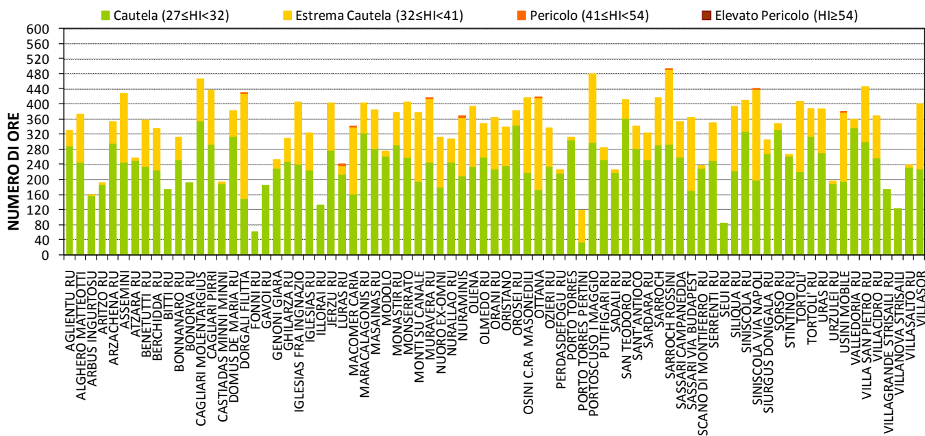
Figura 3. Totale ore mensili con HI nei diversi livelli di disagio – Luglio 2018.
