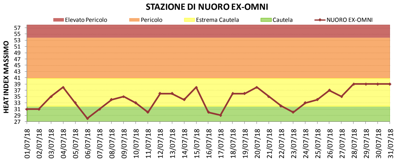
Figura 9. HI massimo giornaliero – Stazione di Nuoro ex-Omni.
